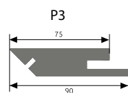
lišta rohová 21x90 délka: 2600 mm
