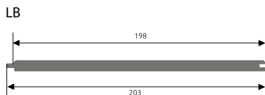
profil obložení 7x203 délka: 2050 mm
