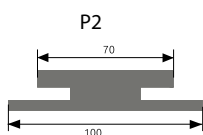
lišta spojovací délka: 2600 mm
